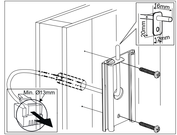
Fig 16: Ledningsdragning genom vägg.
