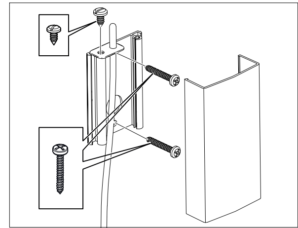
Fig 15: Montering av sensorn
