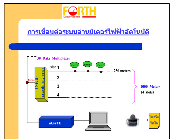
แผนผังการต่อเชื่อมระบบ
